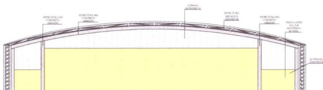
2 FACHADA - FUNDOS GINÁSIO ESCALA 1:125
