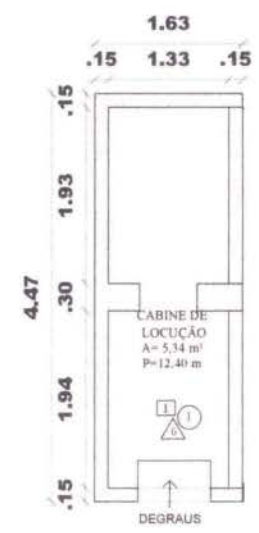
2 PLANTA TÉCNICA ESCALA 1:30
