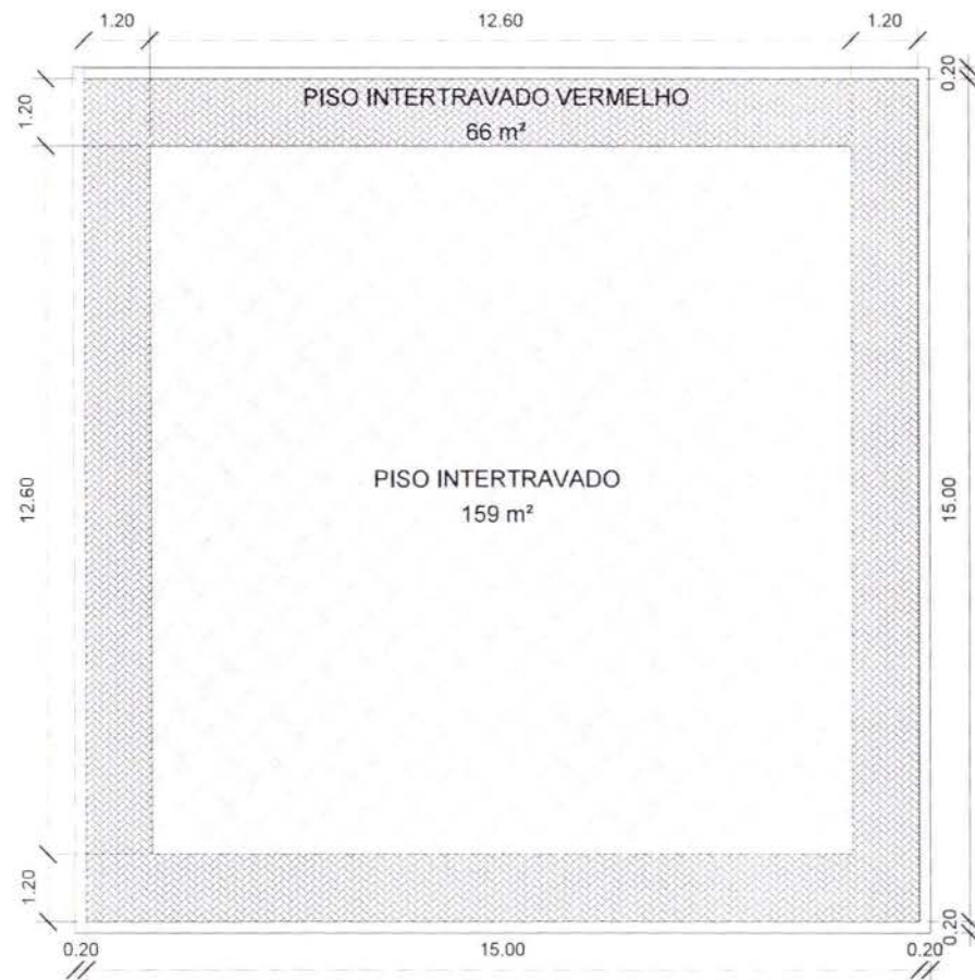
1 PLANTA BAIXA 1 : 100
