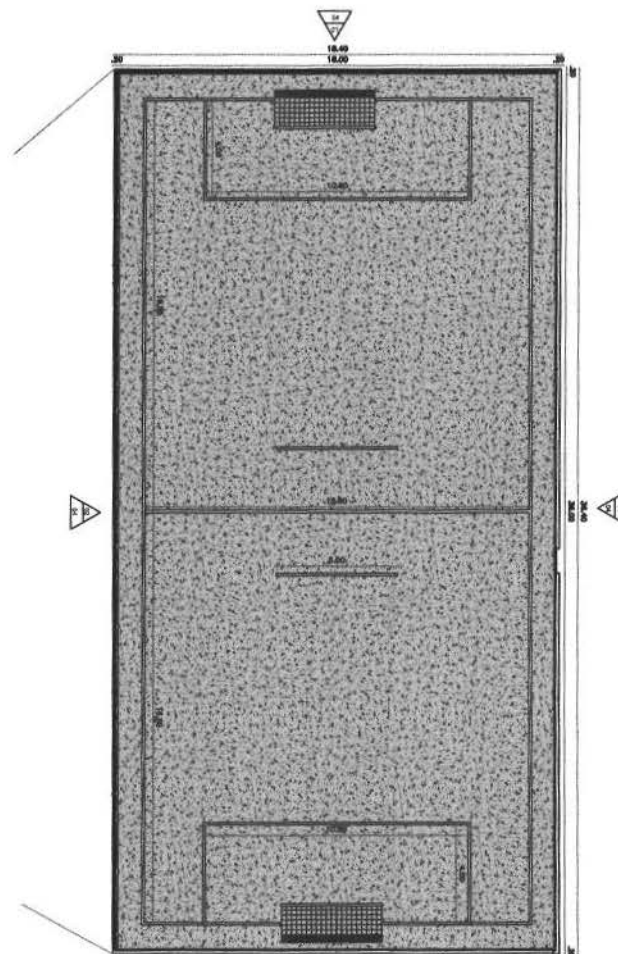
2 PLANTA TÉCNICA - ARENINHA ESCALA 1:50
