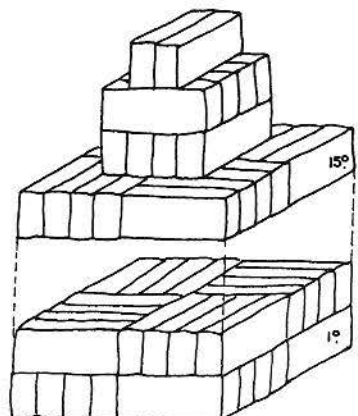
Figura 12 - Empilhamento do tijolo maciço
