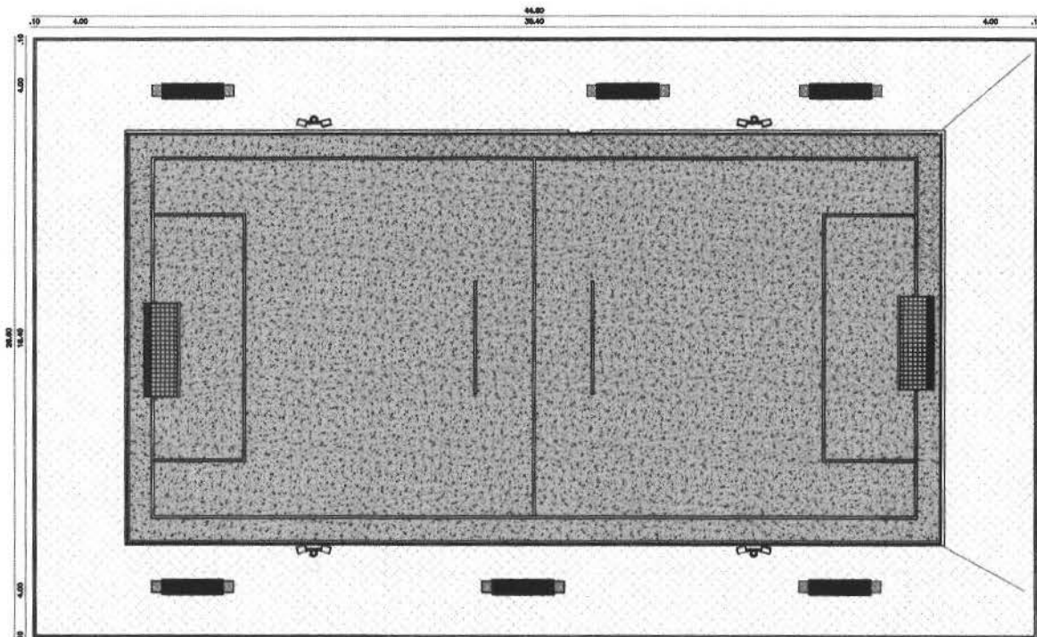
1 PLANTA TÉCNICA ESCALA 1:50
