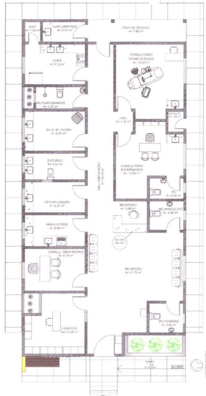
2 PLANTA DE LAYOUT EXPANDIDA ESCALA 1:10
