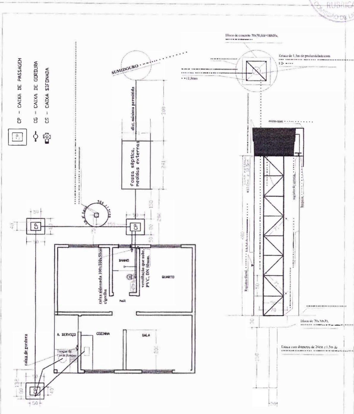
PLANTAS APDID, cx.d'água Esc. 1 / 50
