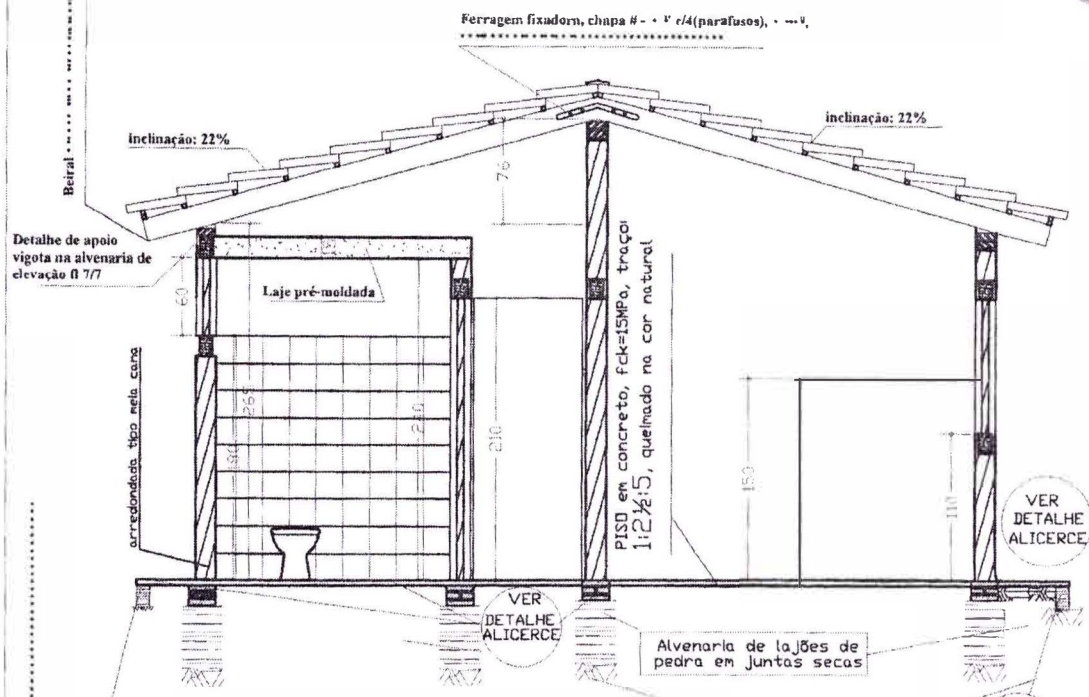
CORTE A-A' (transversal) Esc. 1 / 50
